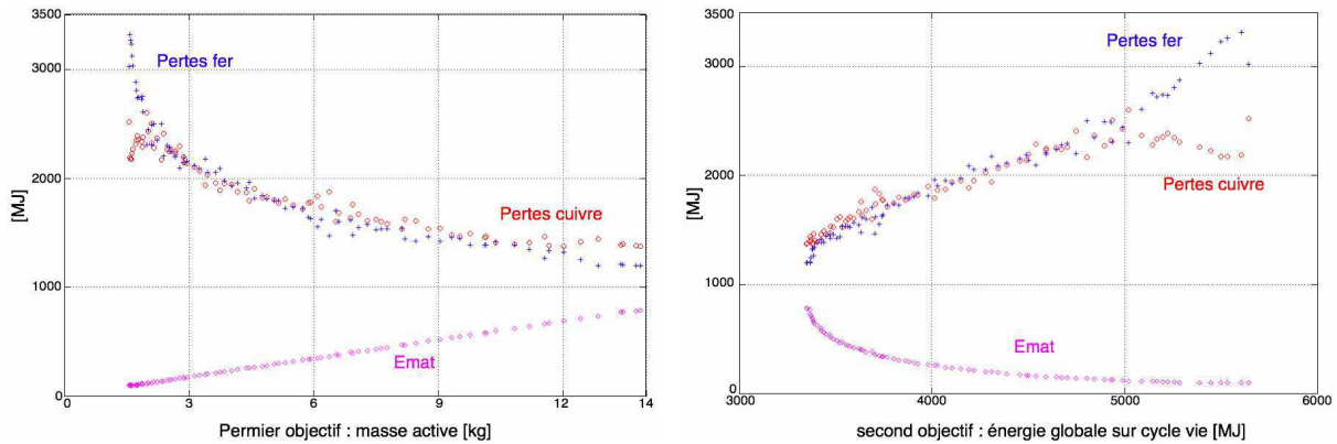
Fig. 7. Répartition des énergies dans E_{LCA} en fonction des deux objectifs sur un profil de charge 12 heures par jour.
