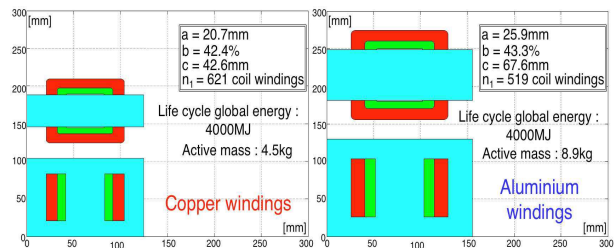
Fig. 12. Comparaison des optimisation sur un même profil de charge de deux matériaux de bobinage différents (ci-dessus) et exemple de solutions à E_{LCA} identiques (ci-contre).
