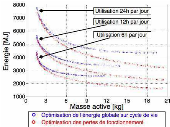
Fig. 6. Transformateur de 230VA. Comparaison de résultats d'optimisation.
