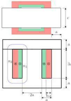
Fig. 3. Paramètres géométriques du transformateur [7].
