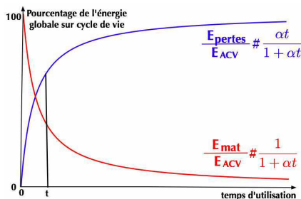
Fig. 8. Contributions énergétiques dans E_{LCA} en fonction du temps d'utilisation. ( \alpha = P_{pertes}/E_{mat} )
