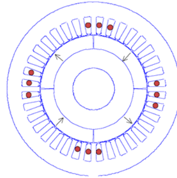
Figure 19. Architecture de principe du générateur : machine synchrone à champ radial, à couplages polaires et à aimants en surface
