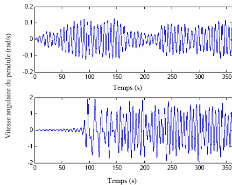
Figure 17. Vitesse angulaire du pendule sans écrêtage (a) et avec écrêtage (b) pour \alpha = 0.8 .
