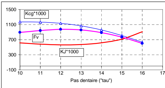
Fig. 9 : Influence du pas dentaire relatif
