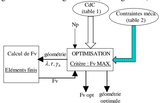
Fig. 13 : Organigramme d'optimisation
