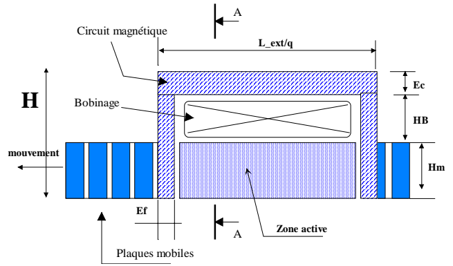
Fig. 4 : Dimensions extérieures largeur extérieure = L_g
