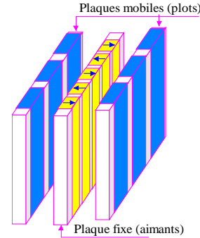
Fig. 6a : Composition des plaques
