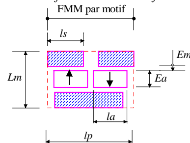
Fig. 6c : Paramètres dimensionnels du motif élémentaire
