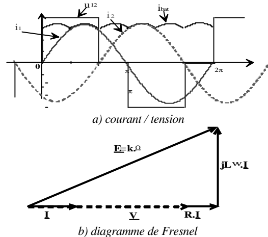
Fig.5 : Formes d'ondes et diagramme de Fresnel de l'étude simplifiée.
