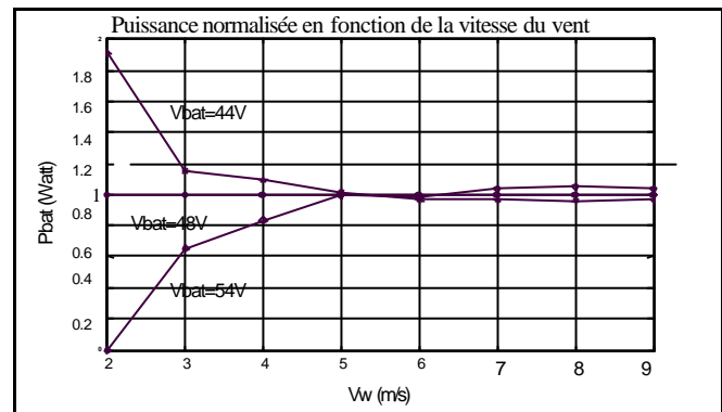
Fig.21 Puissance normalisée fournie par le système en fonction de la vitesse du vent pour plusieurs valeurs de la tension de batterie (étude transfo parfait).
