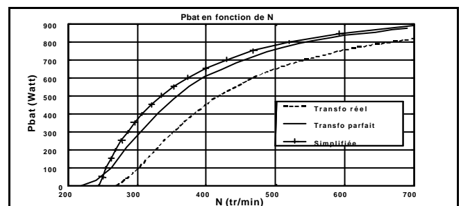
Fig.16 Puissance fournie par le système en fonction de la vitesse pour les trois études.
