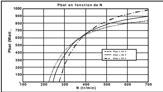
Fig.7 : Puissance en sortie de la chaîne de conversion électrique en fonction de la vitesse de rotation de l'alternateur.
