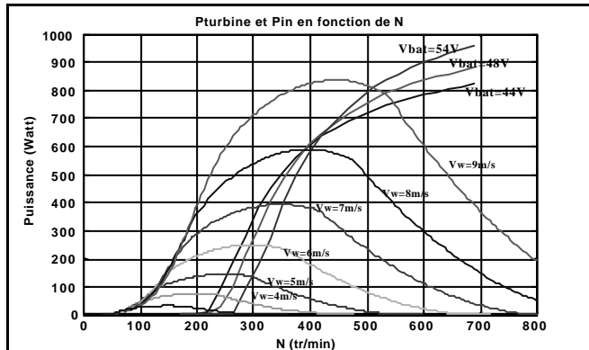
Fig.19 : Puissance fournie par la turbine et puissance en entrée de la chaîne de conversion électrique en fonction de la vitesse de rotation (étude transfo parfait).
