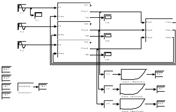
Fig.13 : Schéma Matlab Simulink du transformateur triphasé saturable à 3 colonnes.
