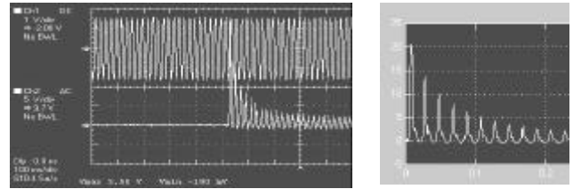
a : tension et courant d'une phase 100V/div, 5A/div, 100ms/div b : courant 5A/div, 100ms/div
