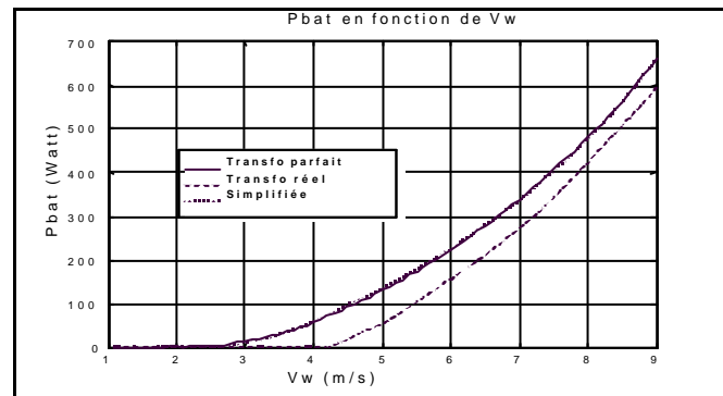
Fig.22 Puissance fournie par le système en fonction de la vitesse du vent pour les différentes études ( V_{bat} = 48V ).
