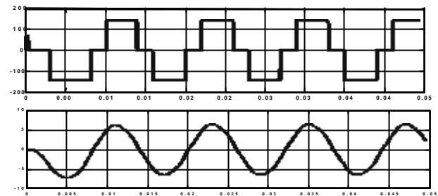
Fig.10 : Tension entre phases et courant dans une phase f=83\text{Hz} , N=622\text{tr/min} , P_{bat}=814\text{W} .
