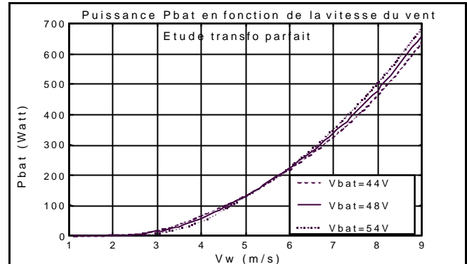
Fig.20 Puissance fournie par le système en fonction de la vitesse du vent pour plusieurs valeurs de la tension de batterie (étude transfo parfait).
