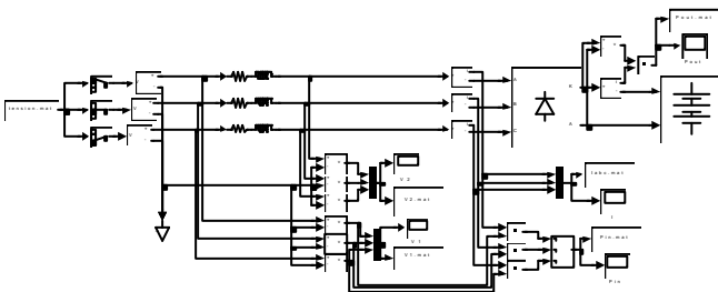
Fig.8 :Synoptique Matlab Simulink – Etude avec Transformateur parfait.
