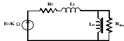
Fig.15 : Schéma électrique équivalent du système transformateur à vide (vents faibles ou secondaire déconnecté).
