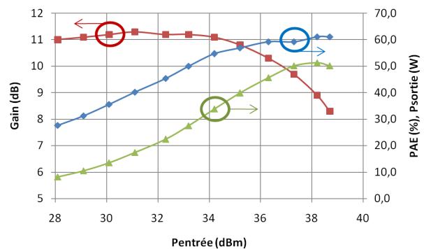
Figure 3. Performances mesurées à 3GHz : Gain (rouge), PAE (bleu), Psortie (vert).
