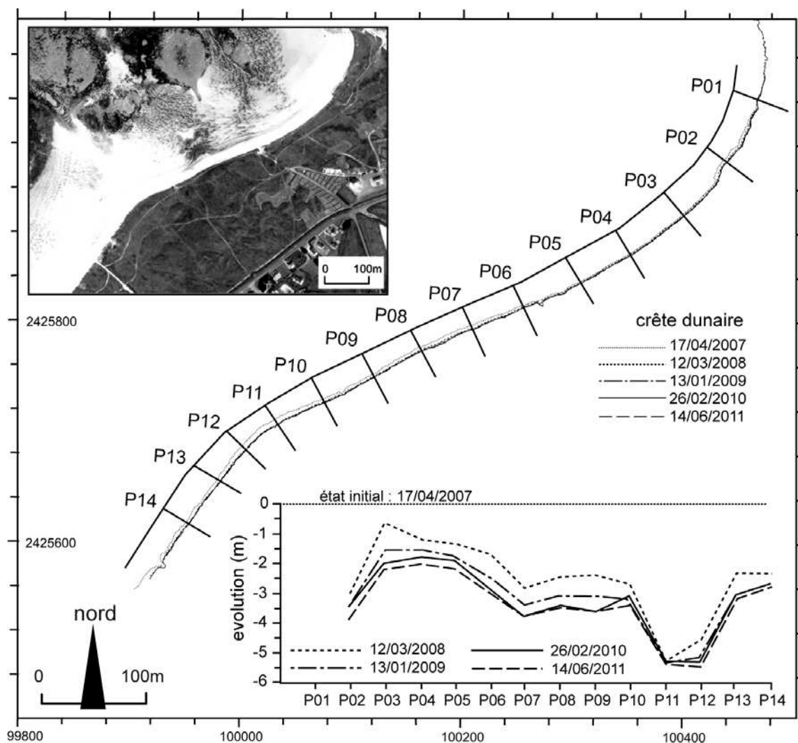
Figure 9 – Cinématique du front de dune entre 2007 et 2011 dans le secteur oriental du cordon dunaire du Vougot
