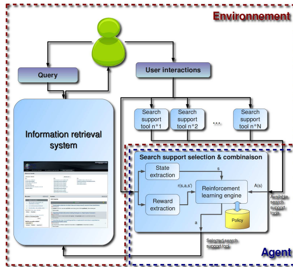
FIGURE 1 – Application du cadre de l'apprentissage par renforcement à la sélection d'outils de support à la recherche.
