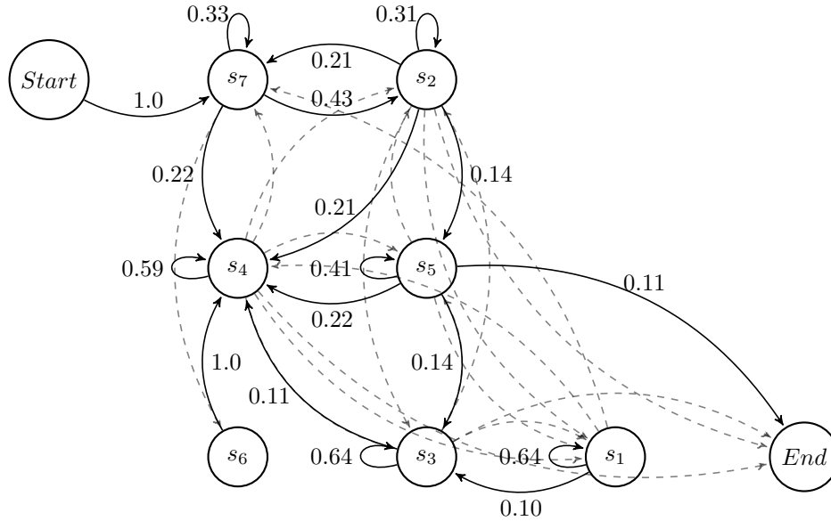
FIGURE 4 – Chaîne de markov donnant les transitions entre 7 états découverts en ignorant les actions (les transitions en pointillé ont un probabilité d’occurrence inférieure à 10%).
