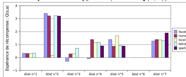
FIGURE 3 – Espérance de récompense “entropyDiff” (valeurs Q(s, a) ) obtenue après apprentissage.
