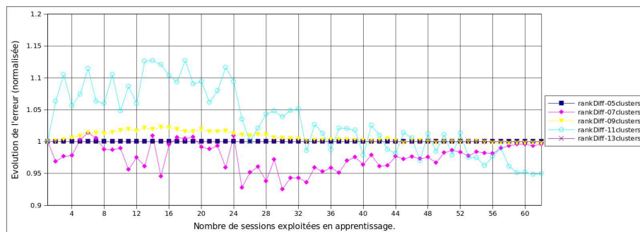
(a) Récompense basée sur le rang des documents manipulés “rankDiff”.
