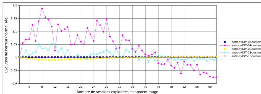
(b) Récompense basé sur la différence d’entropie “entropyDiff”.
