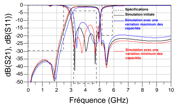
Figure 5. Simulations hybrides de l'étude en sensibilité du filtre
