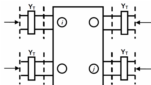
Figure 5. Reconstitution du multipôle avec ses accès
