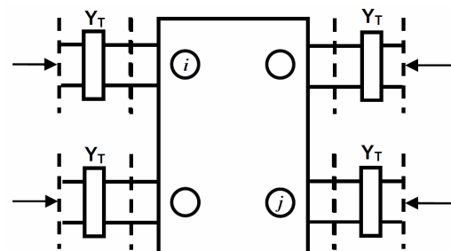
Figure 5. Reconstitution du multipôle avec ses accès
