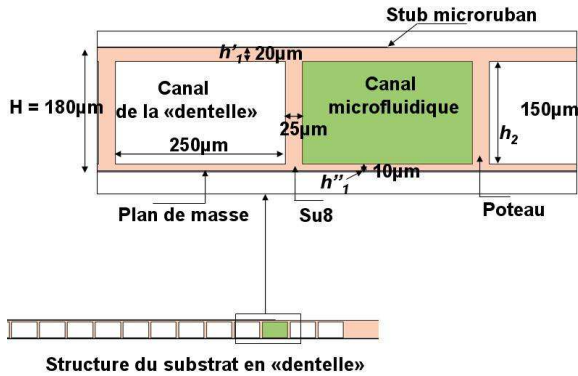
Figure 2. Coupe transversale du substrat évidé
