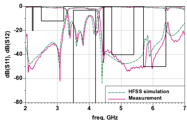
Figure 6. Mesure du prototype et simulation HFSS
