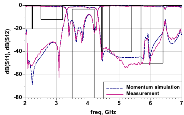
Figure 5. Mesure du prototype et simulation Momentum
