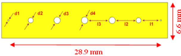
Figure 7. Filtre SIW d'ordre 3
