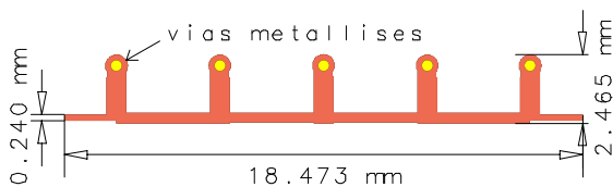
Figure 2. Masque du filtre à stubs CC d'ordre 5.
