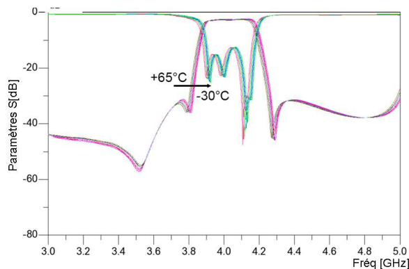
Figure 7. Réponses électriques mesurées du filtre SIW avec boîtier en fonction de la température (-30° → +65°)
