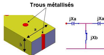
Figure 1. « Coupe » d'un guide d'onde avec des trous métallisés placés au centre avec son circuit équivalent
