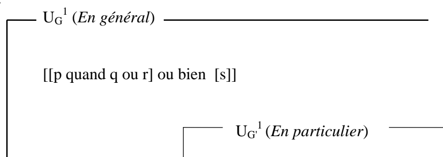
fig.1: installation d'un univers générique U_G^1 , projection d'un univers spécifique parent U_G'^1 , intégration de la séquence [[p \text{ quand } q \text{ ou } r] \text{ ou bien } [s]] sous U_G^1
