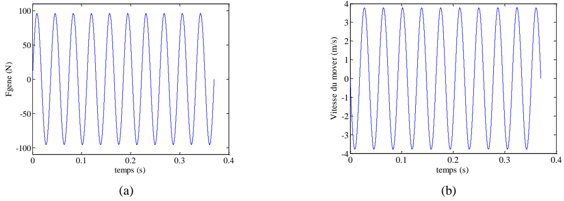
Figure 8 : Allures de la force récupératrice F_{gene} (a) et de la vitesse de déplacement du mover (b)
