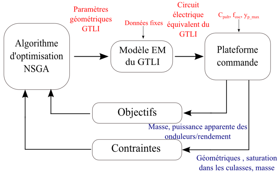
Figure 3 : Synoptique d'optimisation
