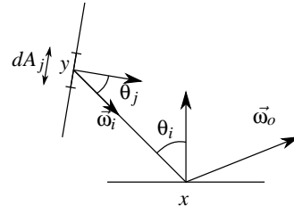
Figure 5: Notations pour l' quation de radiosit .
