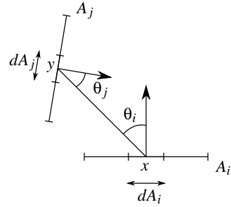
Figure 6: Notations pour l' quation de radiosit  constante discr te.
