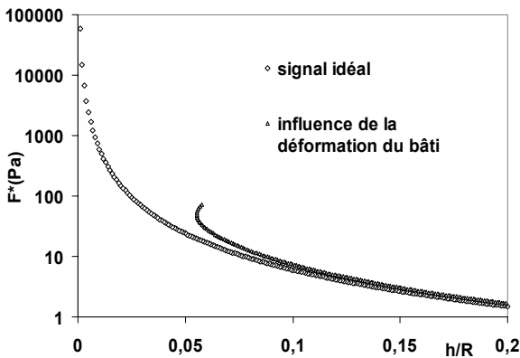
Figure 7 : Influence de la déformation de l'analyseur de texture sur la courbe caractéristique d'un signal idéal newtonien
