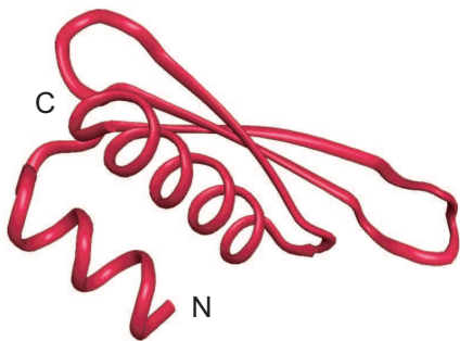
ADAR2 dsRBD1
