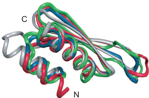
ADAR2 dsRBD1
