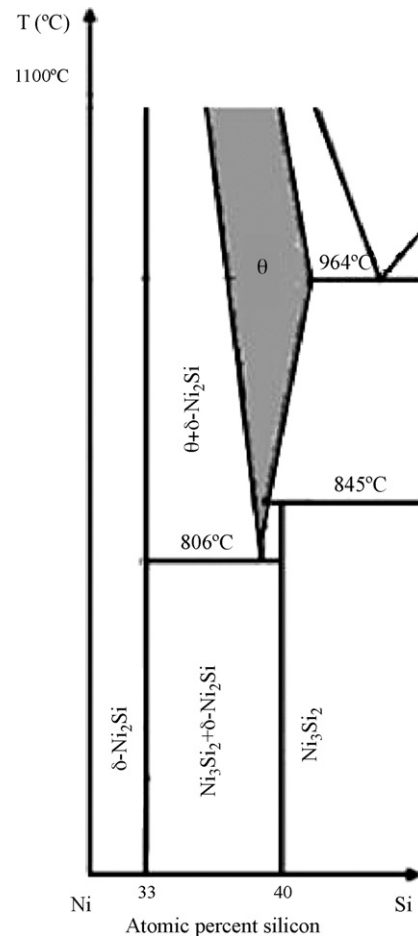
Fig. 4. Ni–Si equilibrium phase Diagram 10 .
