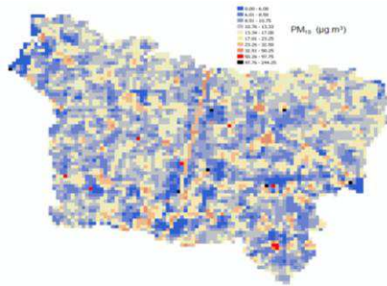
Figure 3 : Cartographie des concentrations en PM 10 en Picardie (en µg.m -3 ).
