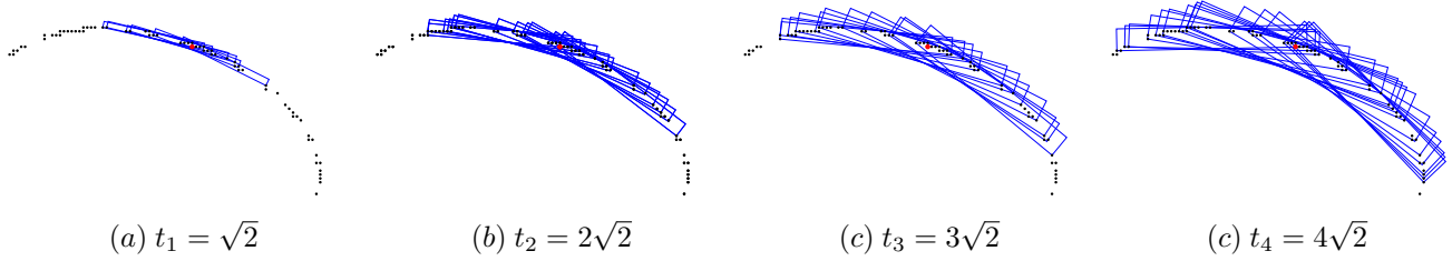
FIGURE 3 – Couverture d’un point par un ensemble de segments flous obtenus à différentes épaisseurs ( t_i ). Pour chaque épaisseur le segment flou couvrant le point considéré (dessiné en rouge) est représenté par des rectangles bleus.
