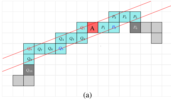
FIGURE 2 – Illustration d’un segment maximal de caractéristiques (a, b, \mu) = (2, 5, 0) , et (b) deux Segments Flous \alpha -épais avec \alpha = 1 (noté 1-épais SF_i avec i = 0, 1 ).
