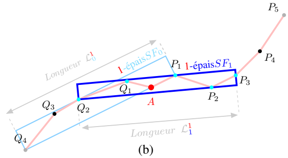
FIGURE 2 – Illustration d’un segment maximal de caractéristiques (a, b, \mu) = (2, 5, 0) , et (b) deux Segments Flous \alpha -épais avec \alpha = 1 (noté 1-épais SF_i avec i = 0, 1 ).
