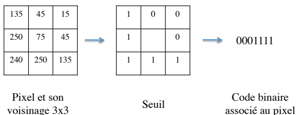
FIGURE 2 – Opérateur LBP.
