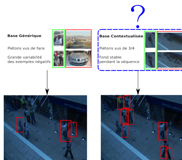
FIGURE 1 – Un classifieur appris sur une base générique (image de gauche) donne de moins bons résultats qu'un détecteur spécialisé (image de droite) lorsque le point de vue de l'ensemble d'apprentissage et celui de la détection diffèrent trop.
