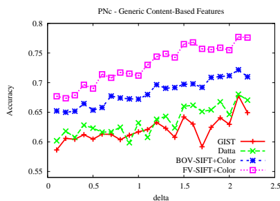
FIG. 3 – Précision sur PnC en utilisant GIST, la combinaison (SIFT+COL) pour les descripteurs BOV et FV.
