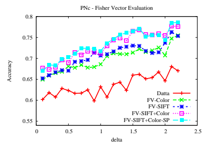
FIG. 4 – Différents FV sur PnC. SIFT et couleur, individuellement, fusionnés, avec la pyramide spatiale.
