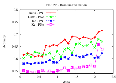
FIG. 2 – Précision pour les descripteurs Datta et al. [25] et Ke et al. [12], évaluée sur PN et PnC (sans les cadres).
