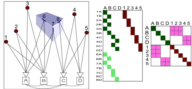
FIGURE 2 – A gauche : un exemple d'ajustement de faisceaux contraint par segments. En rouge foncé, les points 3D de la partie inconnue de l'environnement (1 – 5); en bleu foncé, les segments 3D associés à la partie connue de l'environnement (6 – 8). Les carrés (A-D) représentent la trajectoire de la caméra. Les lignes noires indiquent l'observabilité d'une primitive 3D (point ou segment) à partir d'une certaine pose de la caméra en mouvement. A droite : les matrices Jacobienne et Hessienne associées.
