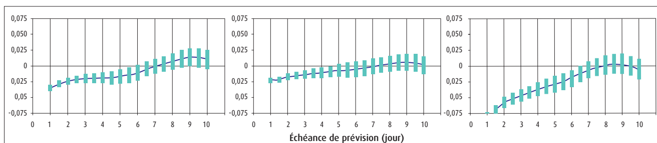
Figure 6 - Apport des spectromètres infrarouges à la prévision numérique dans l'hémisphère sud. L'ordonnée représente la différence de corrélation d'anomalie à 500 hPa entre une prévision avec assimilation des données de Iasi (resp. Airs, resp. Iasi + Airs) et une prévision de référence n'assimilant pas ces données. Les impacts positifs sont indiqués par les valeurs négatives. Avec Iasi, cet impact se fait sentir jusqu'à 6 jours. L'utilisation des deux sondes apporte une amélioration significative du score (jusqu'à 7 jours).
