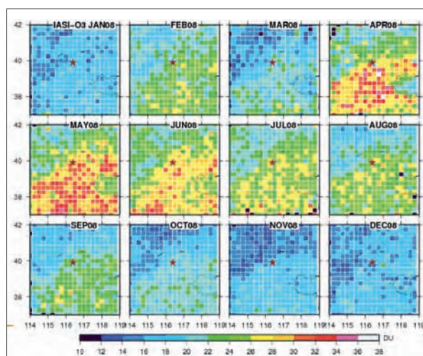
Figure 10 - Distribution spatiale mensuelle de l'ozone de la basse troposphère retrouvé avec Iasi autour de Beijing (Chine). Les valeurs en rouge correspondent à de fortes concentrations. Celles-ci peuvent être observées à partir du printemps lorsque la photolyse devient importante dans les zones à forte concentration urbaine (Dufour et al, 2010).
