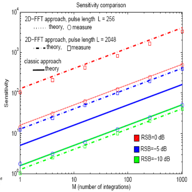
Figure 5: Comparaison des sensibilités pour les 2 procédures ( N=256 ). 3 SNR ( 0\text{ dB} , -5\text{ dB} , -10\text{ dB} ) et 2 longueurs de pulses ( L=256 et L=2048 ) ont été simulés pour différentes valeurs de M (nombre de profils intégrés). Les courbes continues et en pointillé correspondent aux résultats théoriques. Le carrés et les ronds correspondent à la mesure des sensibilités de la méthode FFT 2D/Radon par simulation.
