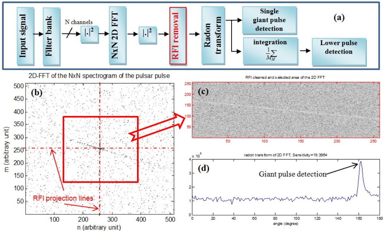
Figure 3: (a) Description de l'algorithme proposé. (b) exemple de la sortie de la FFT 2D 512x512 (l'image a été binarisée pour un meilleure visualisation). les RFIs vont se retrouver projetés sur la croix rouge centrale. La trainée noire correspond à la signature du pulse géant. Cette signature passe systématiquement par le centre de l'image. Seul l'angle change en fonction du DM. (c) Zone centrale extraite de la FFT 2D après élimination de la croix rouge. Cela permet de maximiser la détection (d) Une transformée de Radon permet de mesurer l'énergie présente sur chaque radiale de l'image 3.c. Un pic d'énergie correspond à la présence d'un pulse géant.
