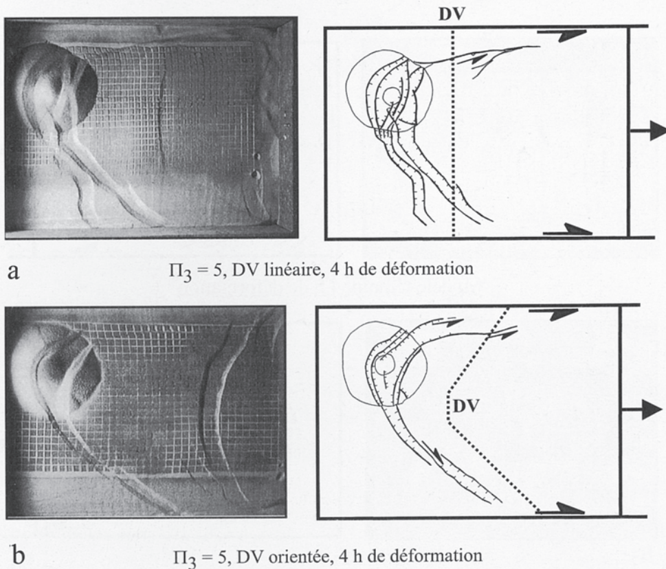
FIG. 7. – Expériences réalisées sur un cône stable gravitairement ( \Pi_3 = 5 ). a : discontinuité de vitesse linéaire ; b : discontinuité de vitesse orientée. Le trait noir représente le trait de coupe.
