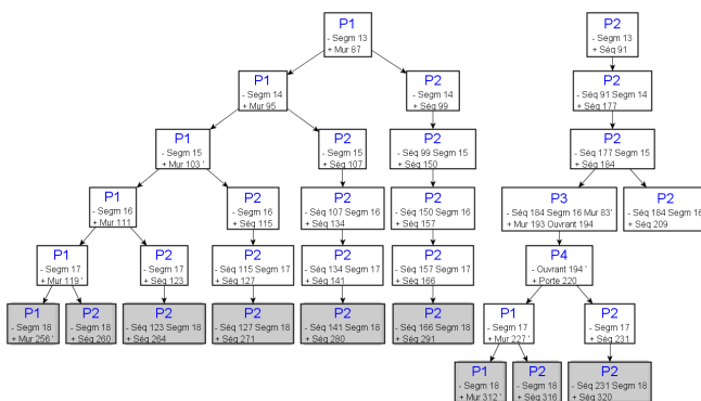
(b) Phase de construction de l'arbre d'analyse de l'étape n+1 (segment 13), déduite de la Figure 5(b). Les nœuds grisés indiquent les nouvelles règles de production appliquées en déplaçant le contexte local.
