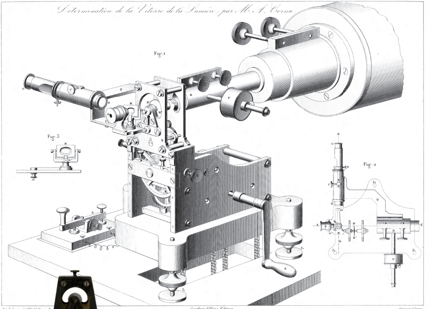
2. Appareil ayant servi à Cornu et Perrotin pour mesurer c. (a) Schéma du dispositif de mesure. La lumière de la lampe (non représentée) passe la roue dentée et entre dans le télescope à droite. La manivelle sert à remonter les poids qui, en tombant, font tourner la roue dentée à travers un engrenage. (Planche issue de la publication d'A. Cornu, Annales de l'Observatoire de Paris : Mémoires, Tome XIII (1876).) (b) Photo de l'appareil. On aperçoit la roue dentée (disque de couleur gris en haut).
