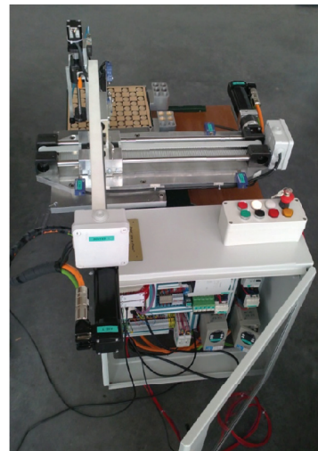
Photo 1 : Le système finalisé
