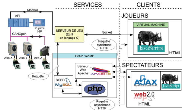
fig. 6 : Schéma de principe de la solution retenue
