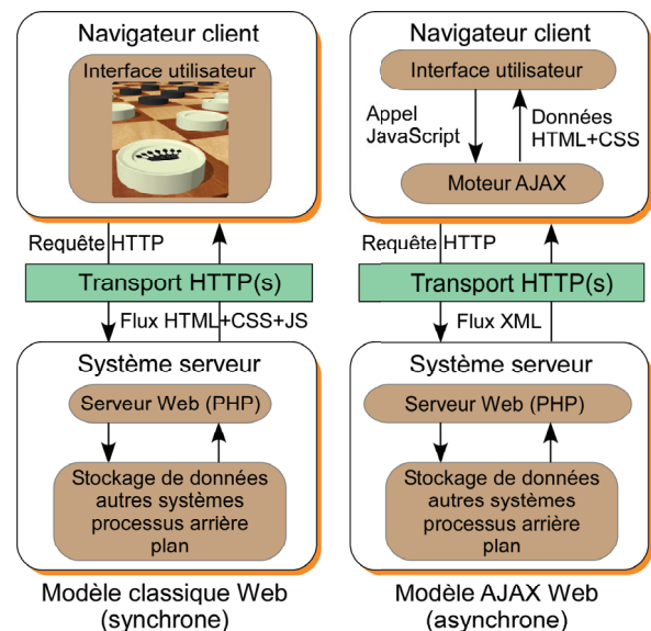
fig. 5 : Les modèles asynchrone et synchrone
