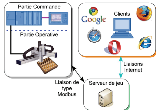
fig. 2 : Vue générale de l'architecture
