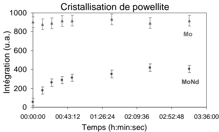
Figure 7. Etude de la cinétique de cristallisation de la phase powellite CaMoO 4 dans les verres Mo et MoNd par DRX HT in situ. Intégration du pic de diffraction de la powellite à 47,05° en fonction du temps, pour une température constante de 750°C. Les deux échantillons ont été broyés et tamisés pour atteindre une taille de particules située entre 80 et 125µm et ont été nucléés (T g +20°C/2h) initialement.
