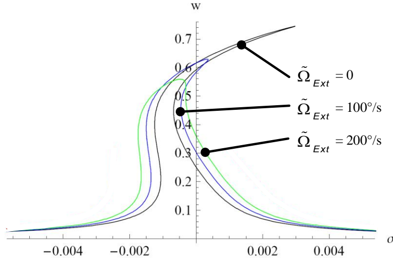
Figure 6. Réponse forcée non linéaire du résonateur ( l = 100\mu\text{m} , b = 5\mu\text{m} , h = 2\mu\text{m} ) quand \tilde{\Omega}_{Act} = \omega_{ms} et pour plusieurs valeurs de vitesse angulaire extérieure.
