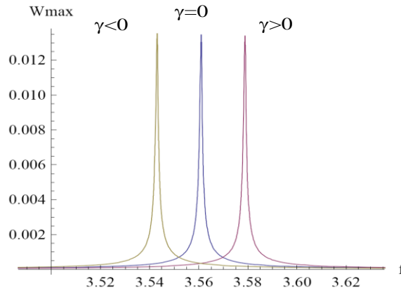
Figure 2. Réponse en fonction de la fréquence d'activation adimensionnée
