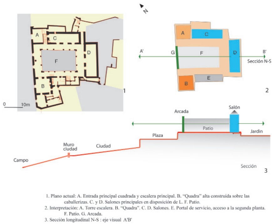
Figura 14 - Palacio de Fuensalida: planta, secciones, restitución.
