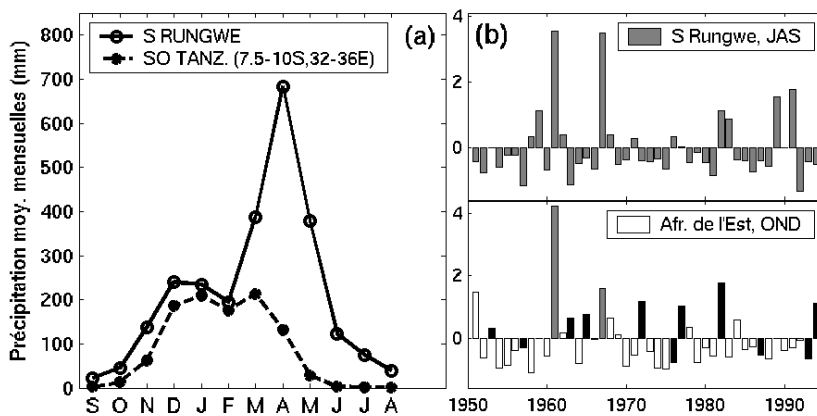
Fig.6 : Précipitations de la région du Mt Rungwe (Tanzanie). (a) Régimes pluviométriques comparés avec les autres stations du sud de la Tanzanie (mm) (b) Evolution des précipitations de Juillet-Septembre (1951-1994) dans la région du Rungwe, et d'Octobre-Décembre en Afrique de l'Est. Barres noires : années El-Nino ; barres grises : années non El-Nino et en même temps anormalement arrosées au Rungwe en juillet-septembre.
