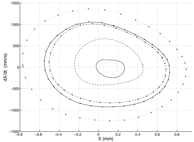
(d) Middle of the brake rod - vertical
