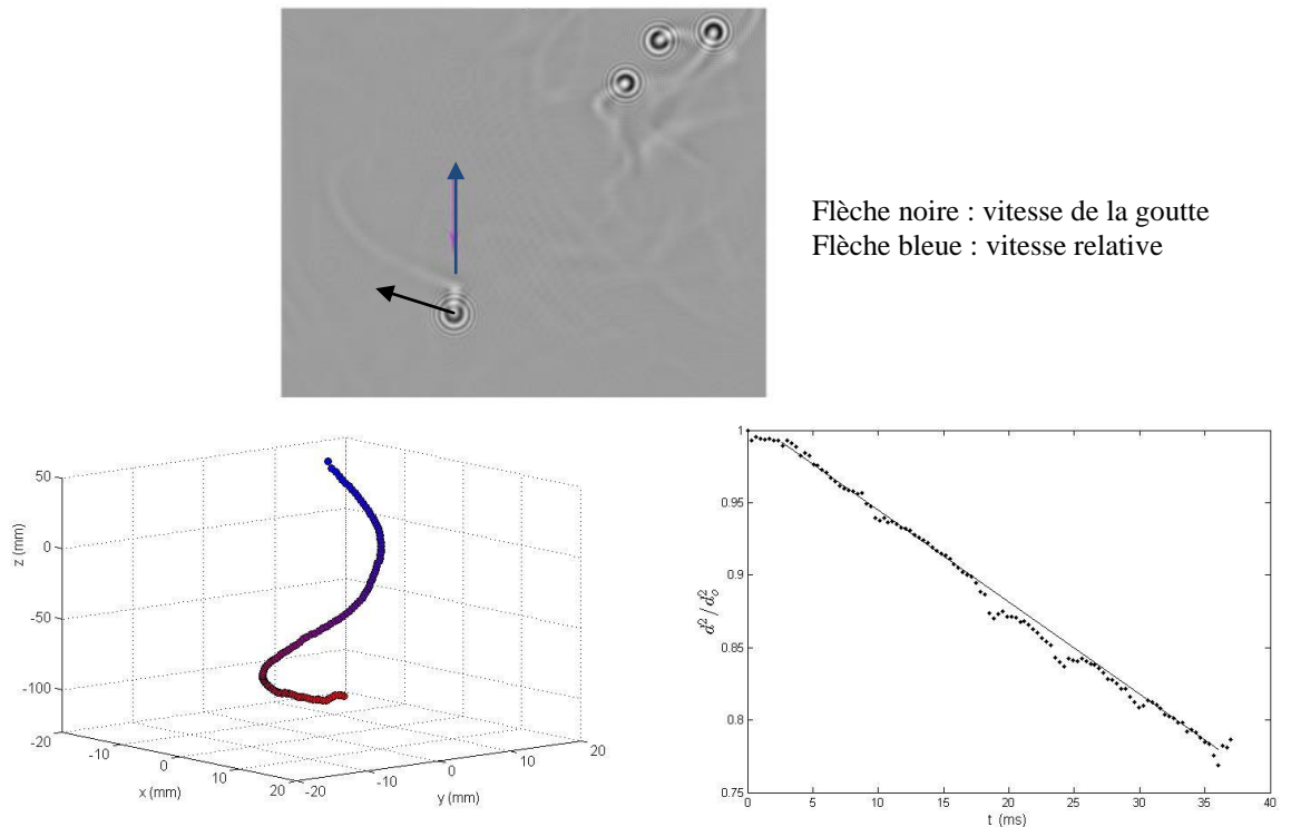
Figure 5: (a) Hologramme de gouttes de fréon (300 µm) ; (b) Trajectoire reconstruite ; (c): Décroissance du carré du diamètre au cours du temps (le long de la trajectoire). 岡岡岡 loi de type Spalding.
