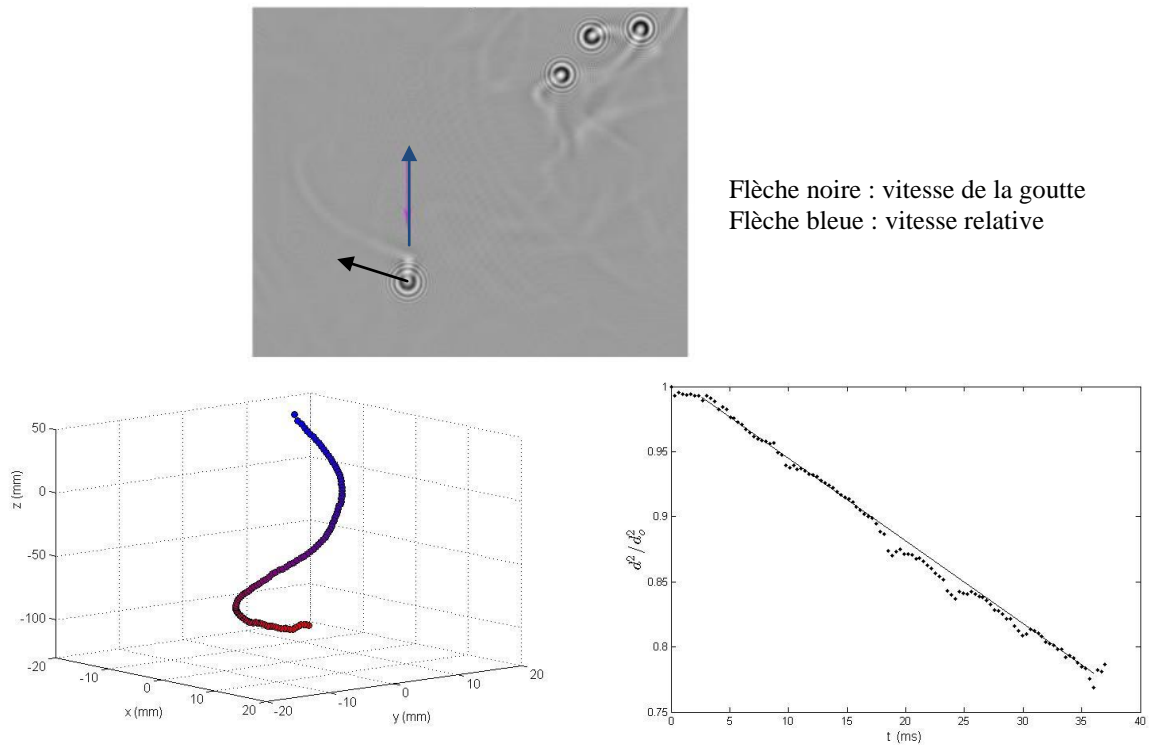
Figure 5: (a) Hologramme de gouttes de fréon (300 \mu m ) ; (b) Trajectoire reconstruite ; (c): Décroissance du carré du diamètre au cours du temps (le long de la trajectoire). loi de type Spalding.
