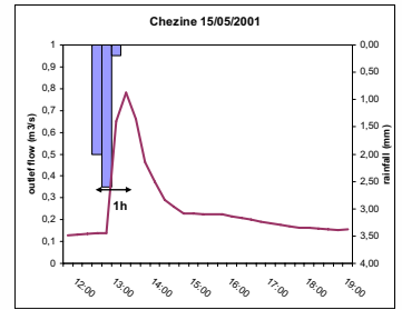
Episode en période sèche: contribution urbaine uniquement: réponse rapide
