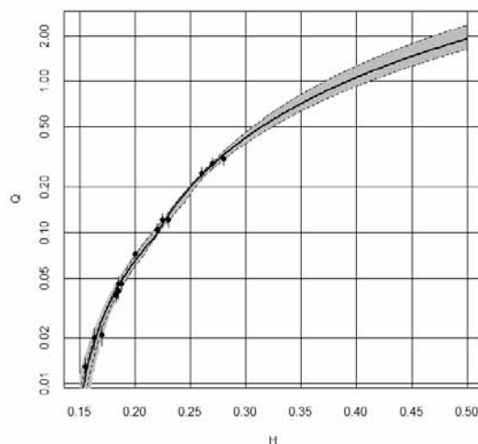
Figure 2 : station du Pont de la Barge sur la rivière Chaudanne (a) et courbe de tarage estimée en échelle logarithmique (b). Les hauteurs sont en m et les débits en m^3/s . En gris l'incertitude sur la courbe représentée par un intervalle de confiance à 95%. Les points sont les jaugeages représentés avec leurs incertitudes respectives.
