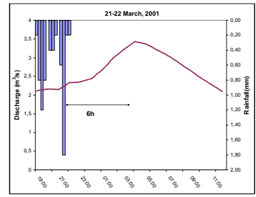
Episode en période humide: contribution rurale importante: réponse lente
