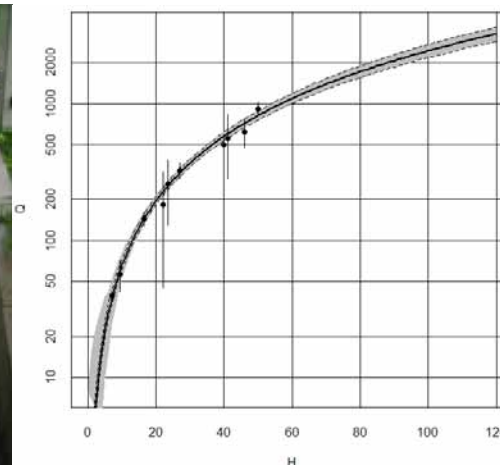
Figure 3 : station de la Léchère sur la rivière Chaudanne (a) et courbe de tarage estimée en échelle logarithmique (b). Les hauteurs sont en cm et les débits en L/s. En gris l'incertitude sur la courbe représentée par un intervalle de confiance à 95%. Les points sont les jaugeages représentés avec leurs incertitudes respectives.
