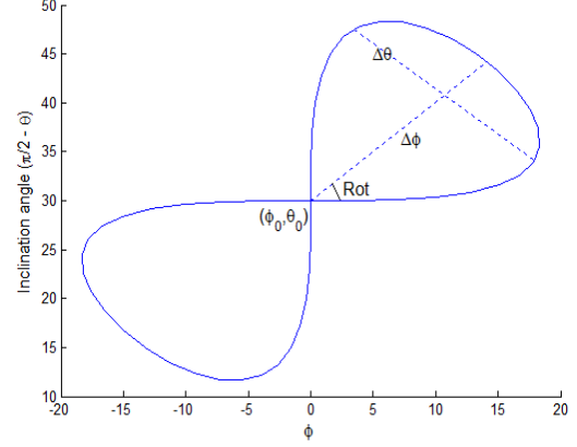
Fig. 3. Orbit parameters.
