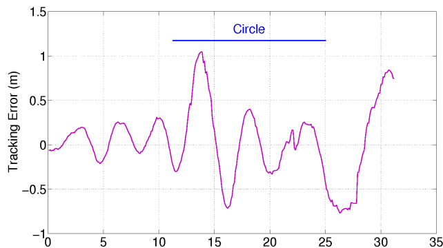
Fig. 9. Tracking error
