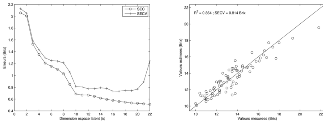
Figure 1 - Étalonage du modèle de mesure du taux de sucres des pommes. À gauche, évolution des erreurs en fonction du nombre de variables latentes de la PLS ; À droite, prédictions de la validation croisée pour k=10 variables latentes.
