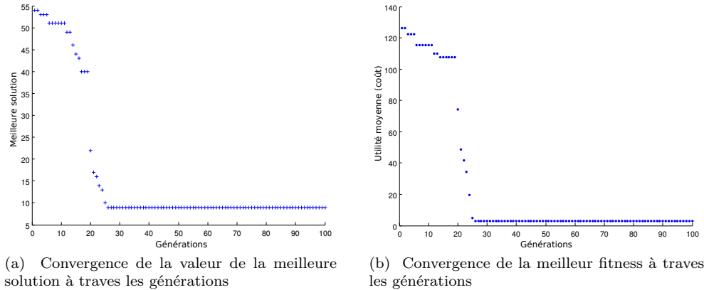
FIG. 6: Convergence de l'AG (à représentation réelle) : optimisation des périodes de maintenance d'un seul composant
