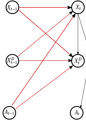
FIG. 1: Structure d'un modèle graphique probabiliste associé à un MGD. Les arcs en gras caractérisent les dépendances temporelles.
