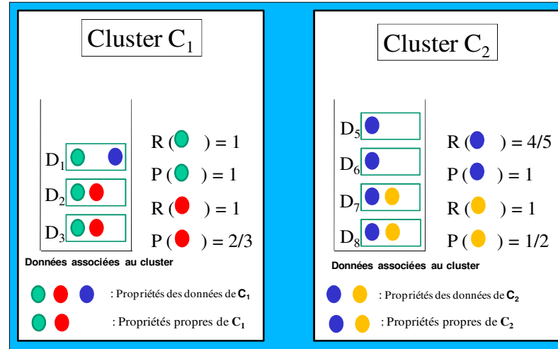
Figure 1. Principe des indices de Rappel(R)-Précision(P) non supervisés.
