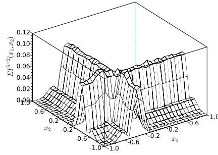
(d) 3D plot of 2 points EI, EI^{(0,2)}(\mathbf{x})
