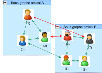
FIG. 1 – Réseau de sources S_1 à S_7 non cohérent et sa partition optimale (lien d'affinité en vert, d'hostilité en rouge).
