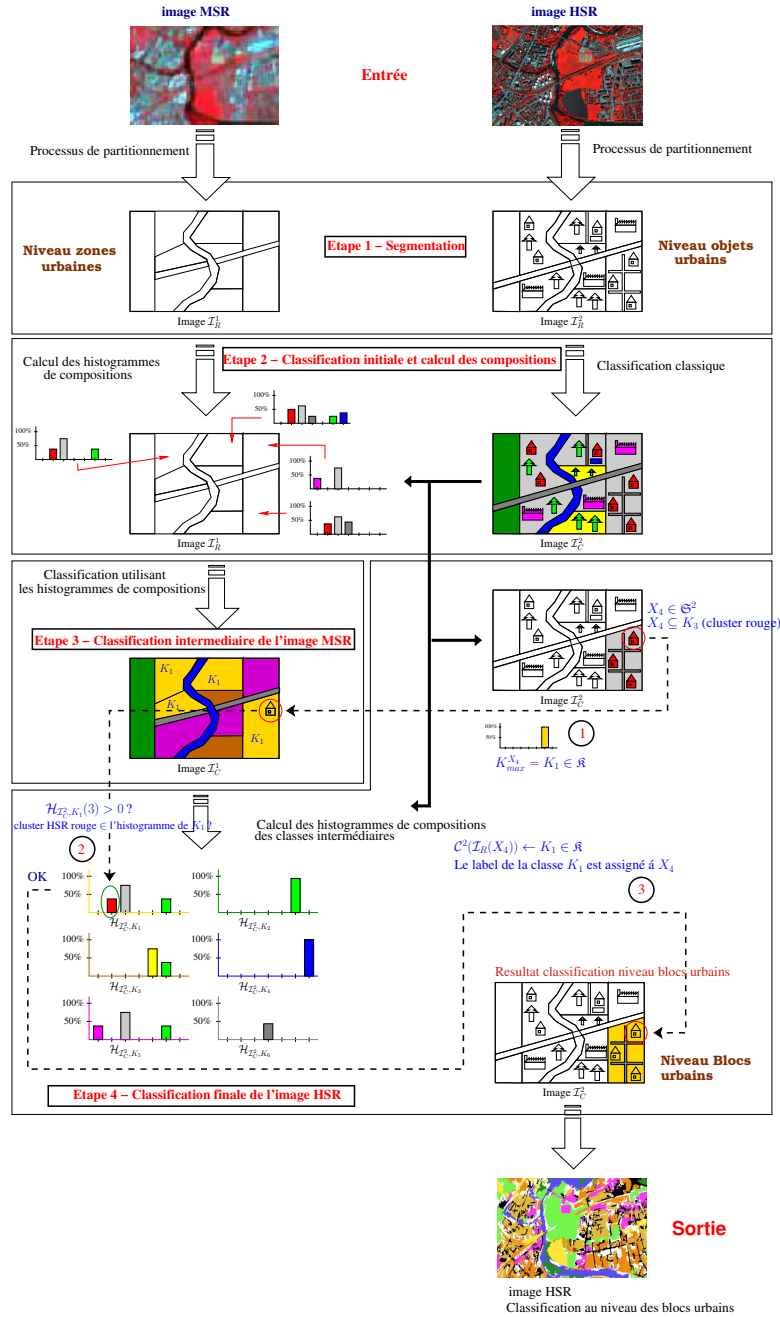
FIG. 2 – Schéma de la méthode proposée : la méthode prend en entrée deux images, une MSR et une HSR, et fournit en sortie une classification de l'image HSR segmentée au niveau sémantique des blocs urbains.
