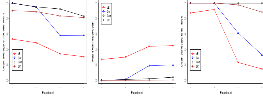
FIG. 4 – Evaluation des métriques pour la classification des profils d’expression simulés. La progression des valeurs moyennes des critères asw (gauche), wbr (milieu) et RI (droite) est illustrée.
