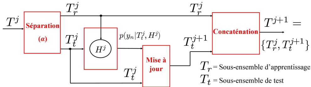
FIG. 1 – Schéma de la procédure itérative améliorée qui permet d'éviter le phénomène de sur-apprentissage.
