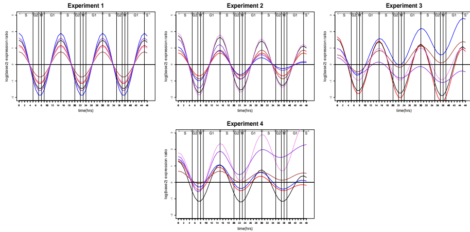
FIG. 3 – Profils des gènes de la phase G_1/S suivant les quatre expériences.
