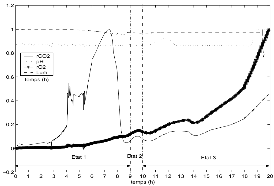
FIG. 1 – Etats physiologiques fournis par les experts sur un bioprocédé de type batch. L'axe des abscisses représente le temps exprimé en heures, l'axe des ordonnées représente l'amplitude des paramètres biochimiques (les valeurs ont été normalisées). 4 paramètres ont été utilisés : le pH, la vitesse de consommation de l'oxygène ( rO_2 ), la vitesse de production de dioxyde de carbone ( rCO_2 ) et la luminance (Lum) qui traduit la production de biomasse. On distingue 3 états : la fermentation (état 1), la diauxie (état 2), l'oxydation (état 3).
