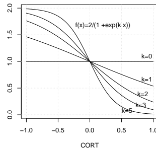
FIG. 1 – L'effet du réglage en fonction de k
