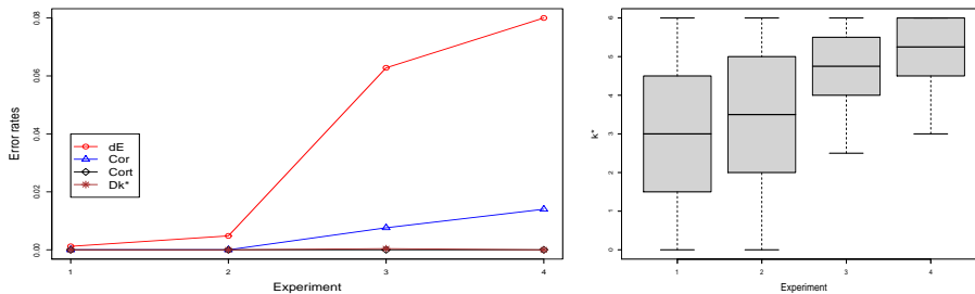
FIG. 5 – Progression des taux d'erreur moyens des classements suivant les expériences (gauche). Distribution de k^* pour les classements adaptatifs suivant les expériences (droite)
