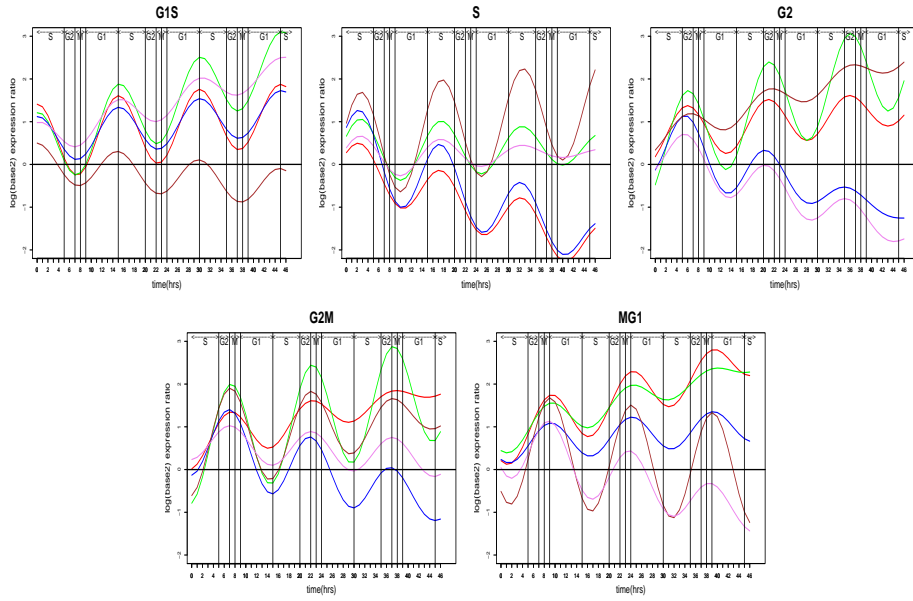
FIG. 2 – Progression de l'expression des gènes durant les 5 phases G_1/S , S , G_2 , G_2/M et M/G_1 .
