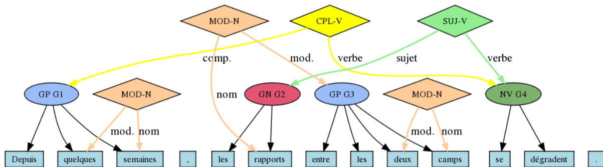
Figure 1. Exemple de sortie au format Passage
