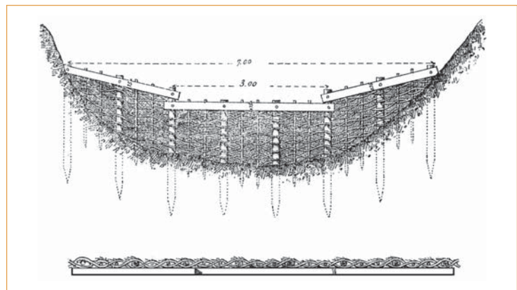
▲ Figure 3 – Barrage en clayonnage de 1 er ordre à 1 parement (Thiéry, 1891).
