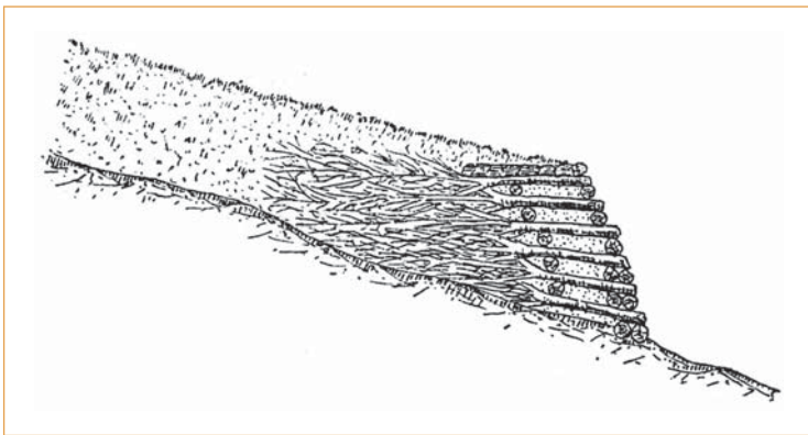
▼ Figure 1 – Barrage en caisson végétalisé (Thiéry, 1891).
