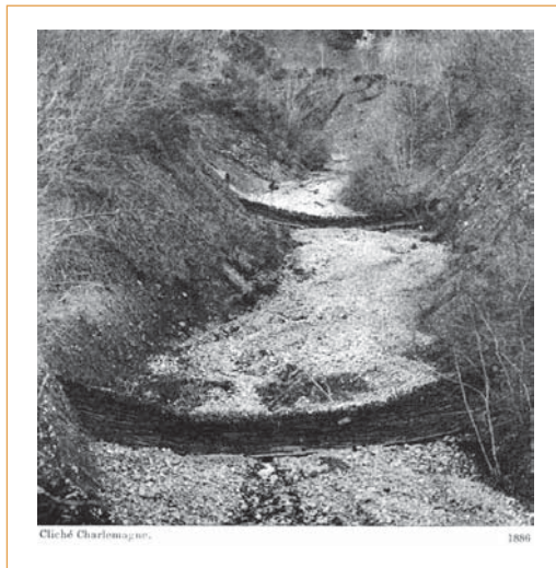
► Figure 4 – Clayonnages dans le torrent de l'Echarina, Isère (Kuss, 1903).
