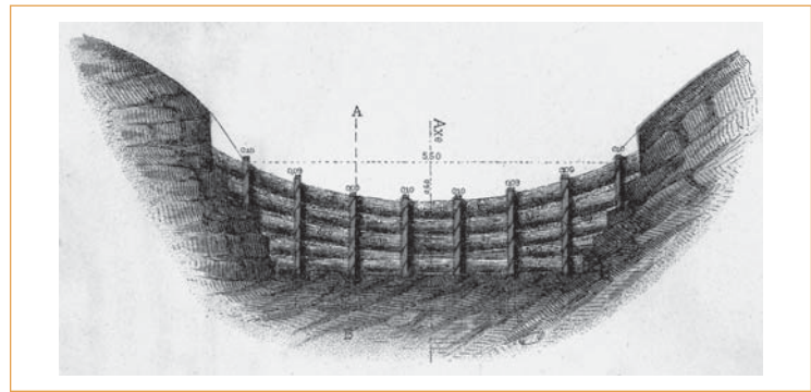
▲ Figure 2 – Barrage en fascinaige de 1 er ordre (Demontzey, 1875).
