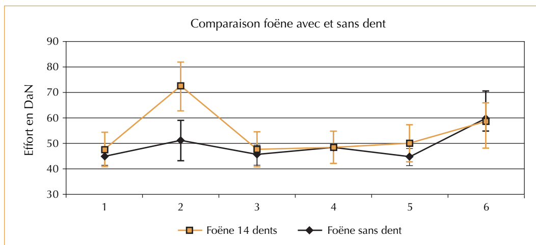
◀ Figure 4 – Courbe d'effort d'extraction des foënes avec et sans dents des 6 tas.
