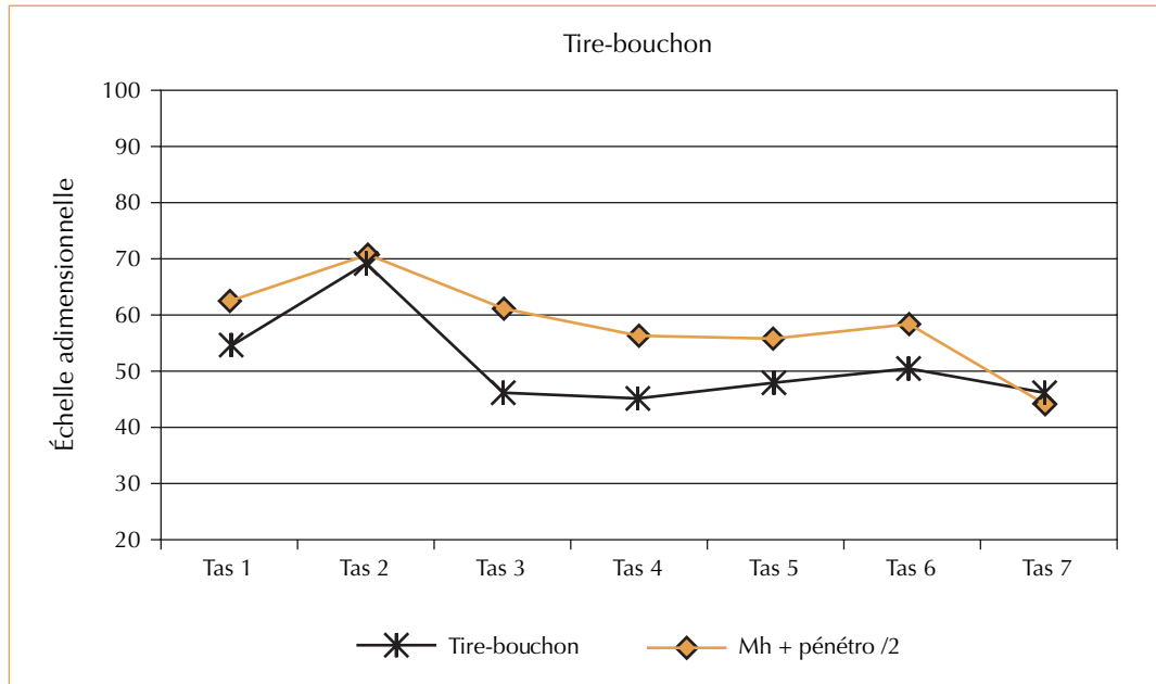
► Figure 2 – Valeurs obtenues avec le tire-bouchon comparées à la demi-somme de mesures classiques.
