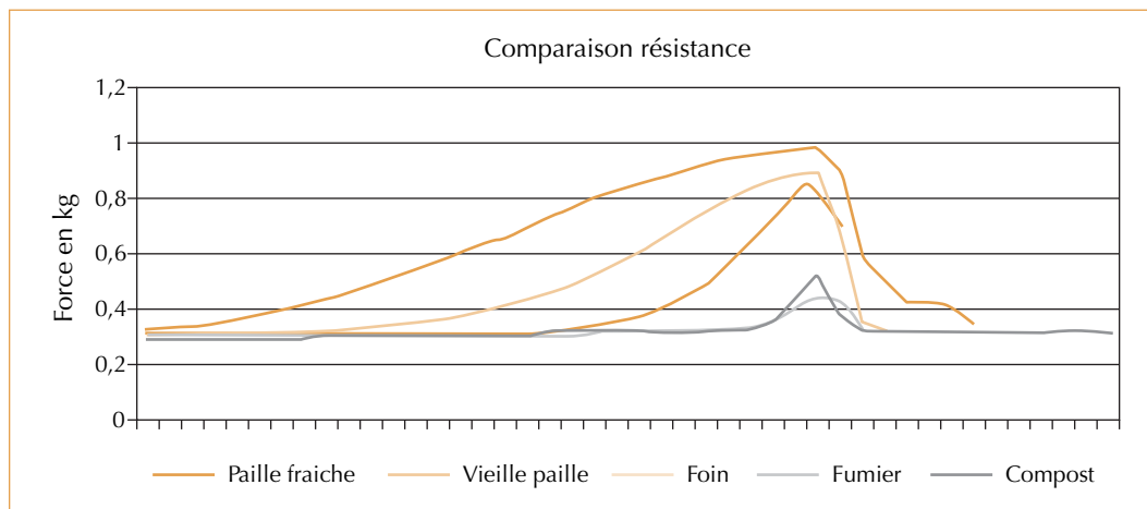
◀ Figure 1 – Influence du vieillissement de la paille sur la force de cisaillement et comparaison avec le foin et des brins extraits du fumier ou du compost.
